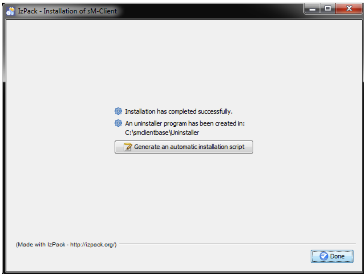
Abbildung 9 Installationsende
