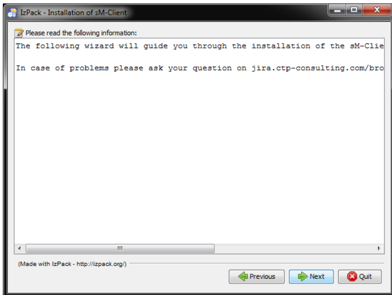
Abbildung 2 Information-Screen
