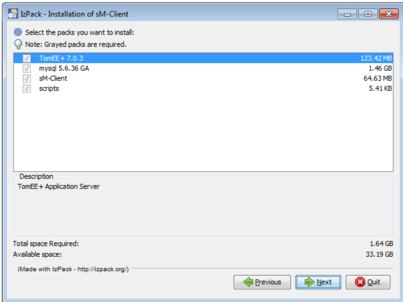
Abbildung 4 Package-Screen
