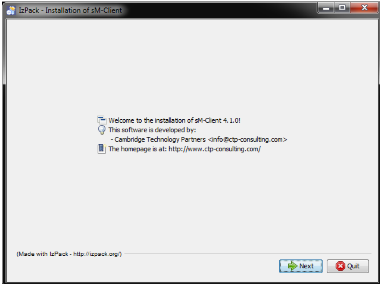
Abbildung 1 Welcome-Screen
